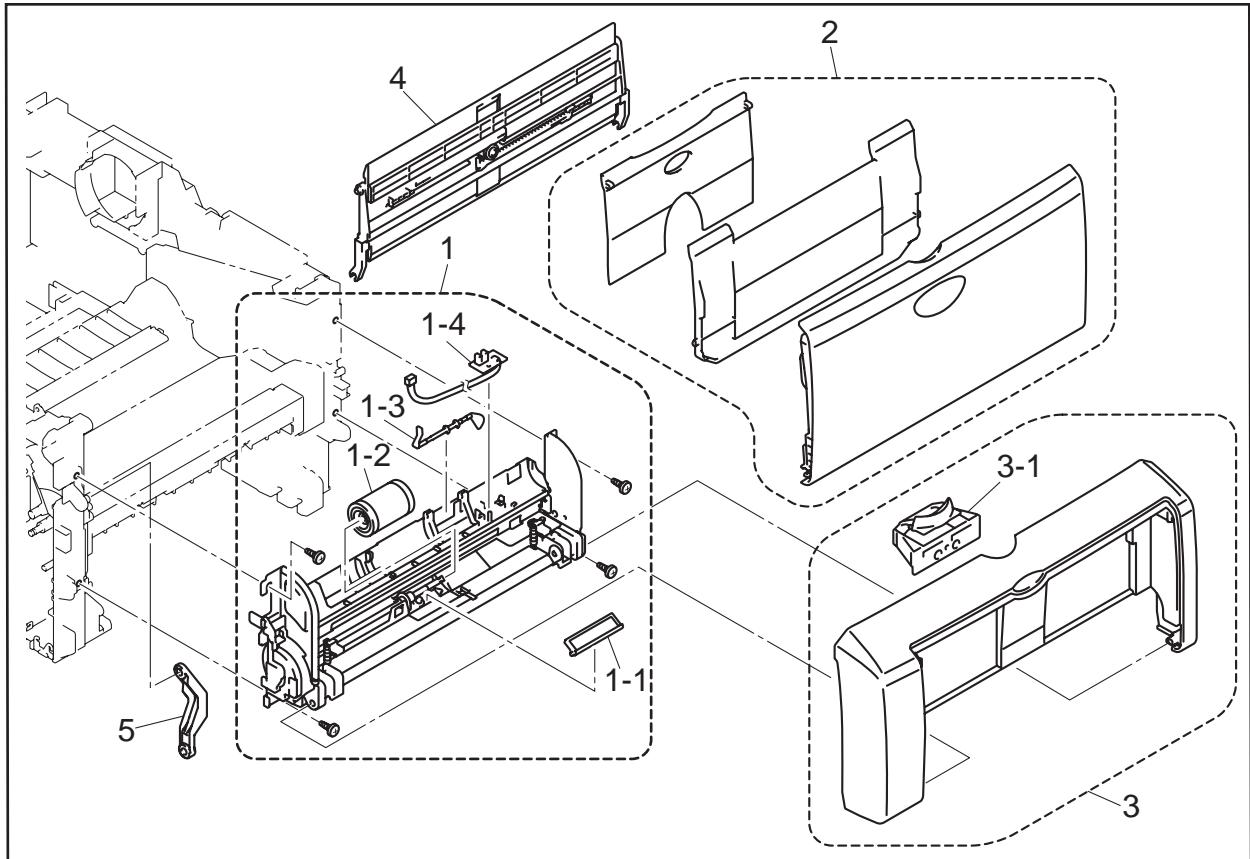
MODEL HL-5050/5070N/5050LT US 84U-Z43/Z44/Z46-041
